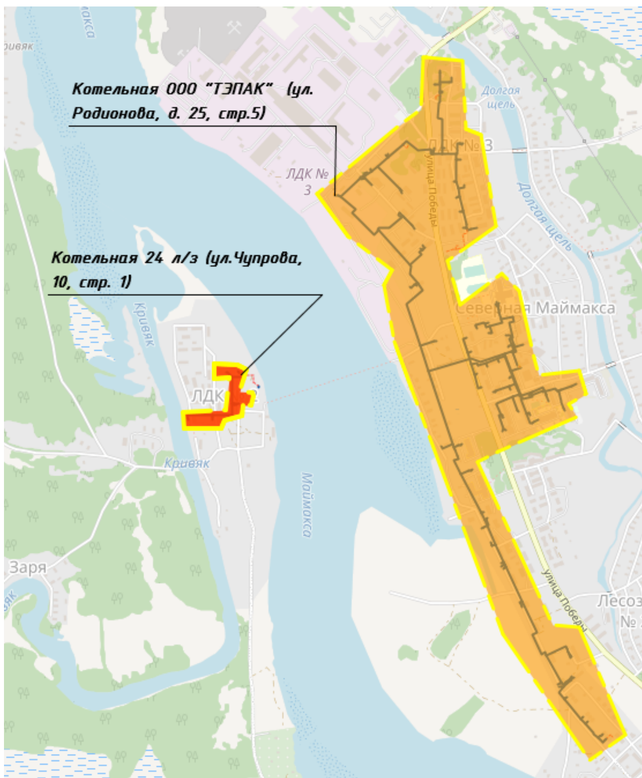
Рисунок 32. Зоны действия котельной ООО «ТЭПАК» ул. Родионова, д. 25, стр. 5 и котельной 24 л/з ул. Чупрова 10, стр. 1
