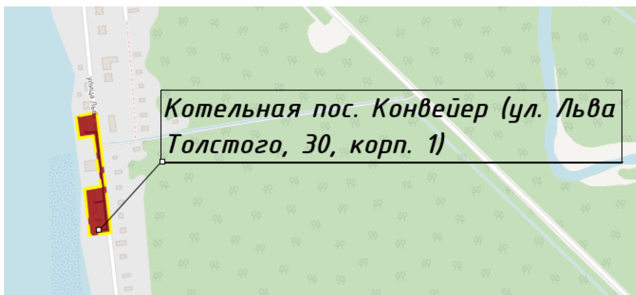
Рисунок 25. Зона действия котельной пос. Конвейер, ул. Льва Толстого 30, корп. 1
