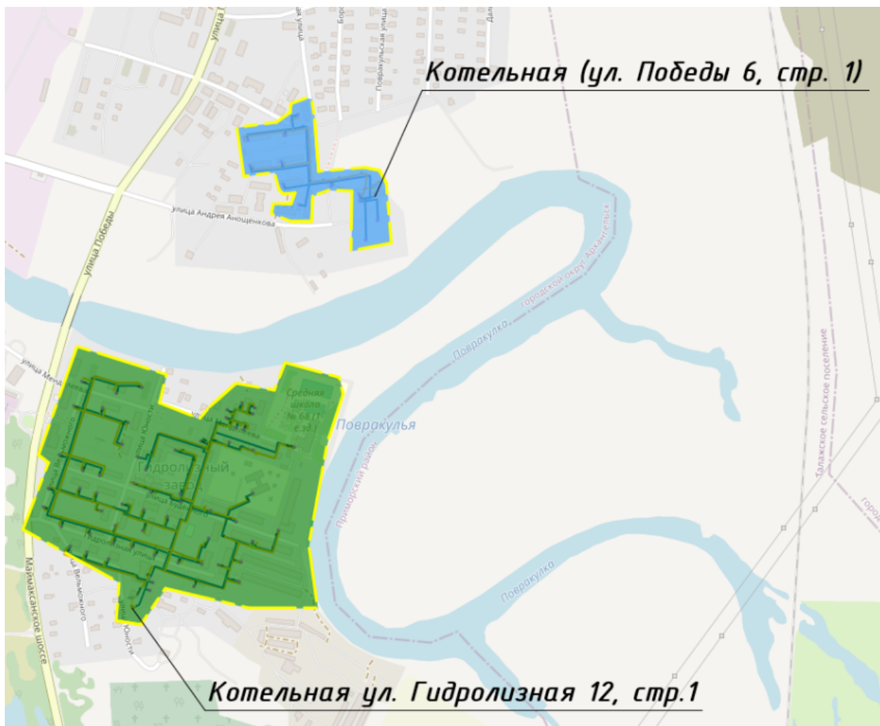
Рисунок 27. Зоны действия котельной ул. Победы 6, стр. 1 и котельной ул. Гидролизная 12, стр. 1
