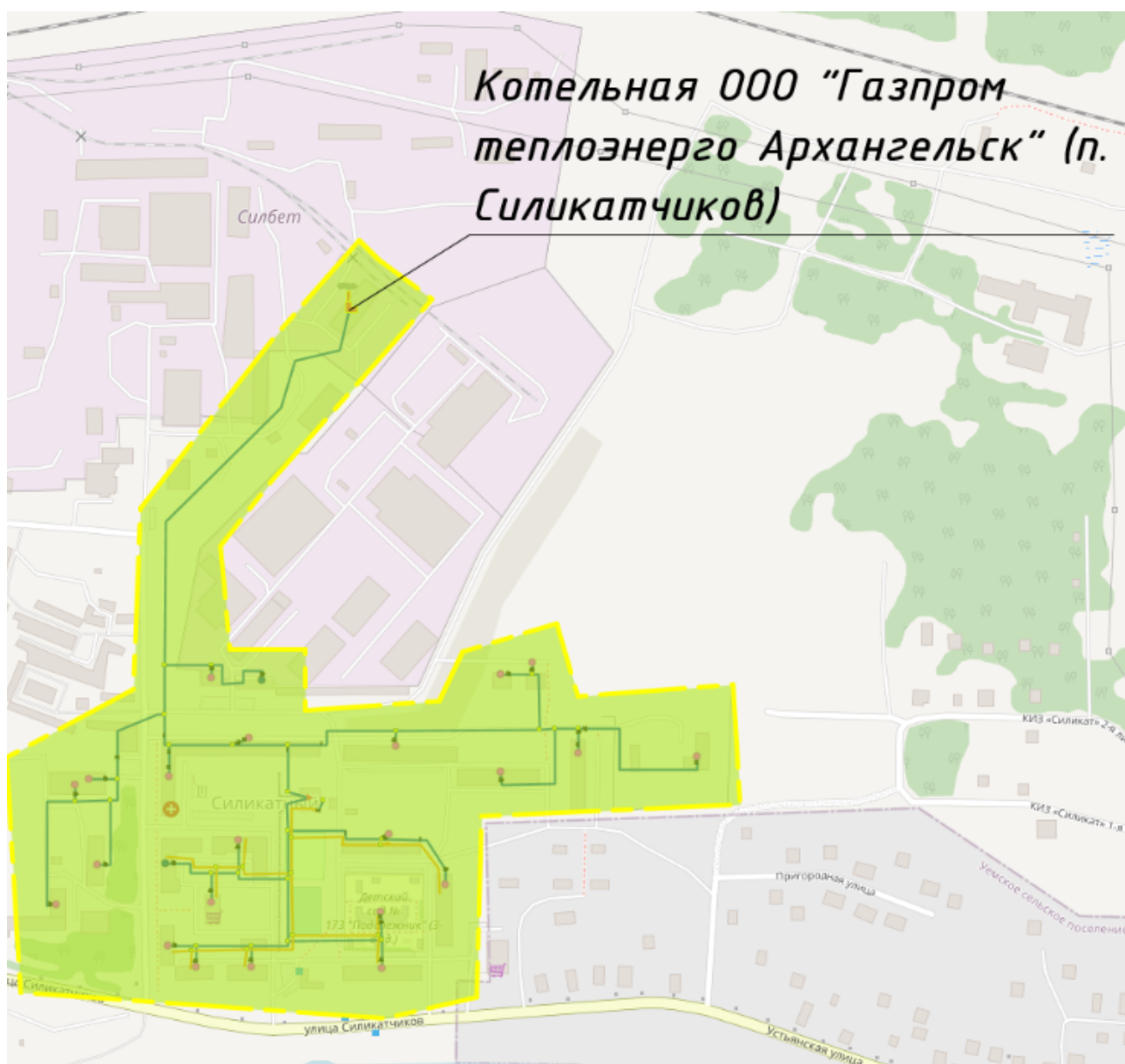
Рисунок 21. Зона действия котельной ООО «Газпром теплоэнерго Архангельск» п. Силикатчиков
