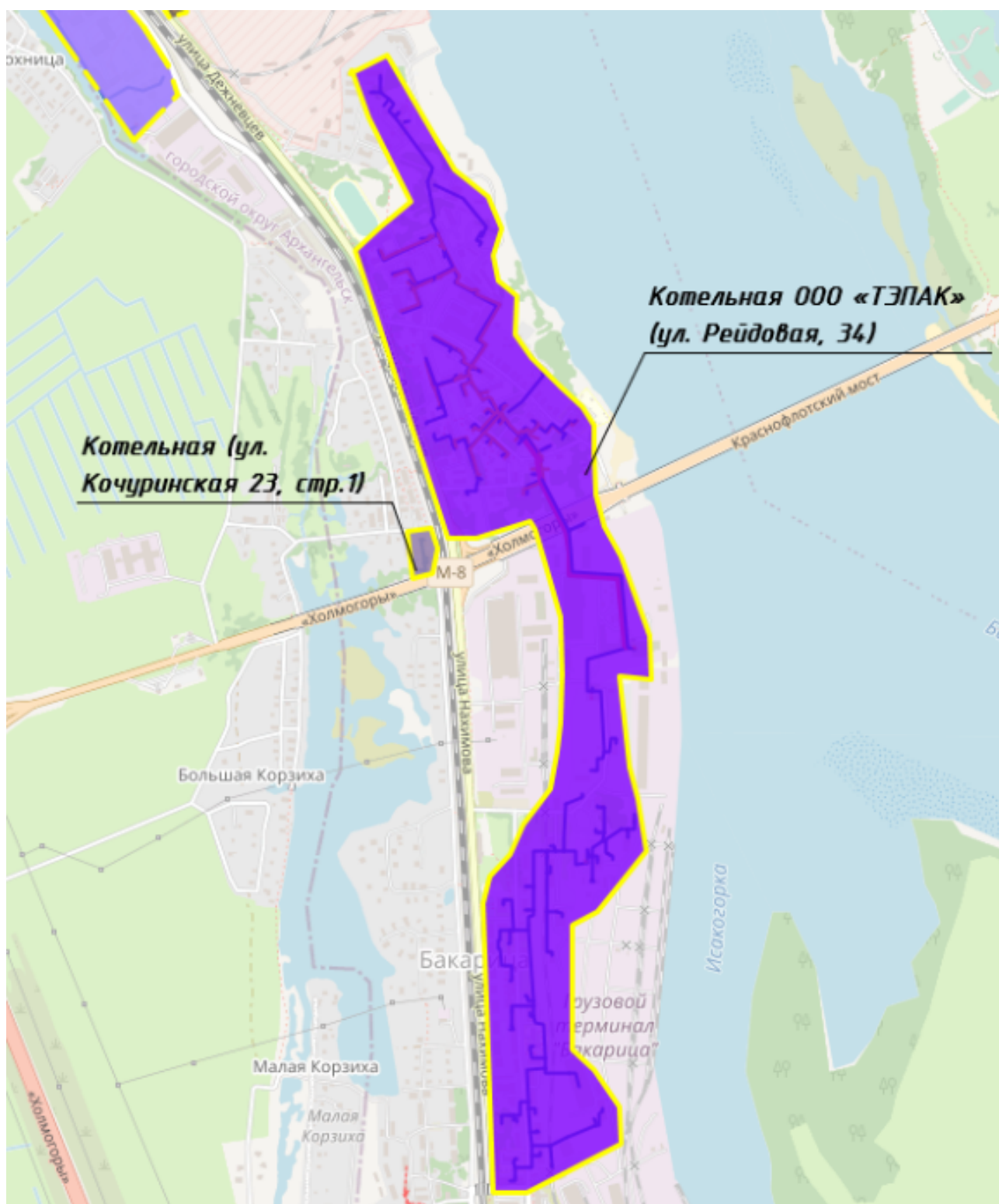
Рисунок 30. Зоны действия котельной ООО «ТЭПАК» ул. Рейдовая 34 и котельной ул. Кочуринская 23, стр. 1
