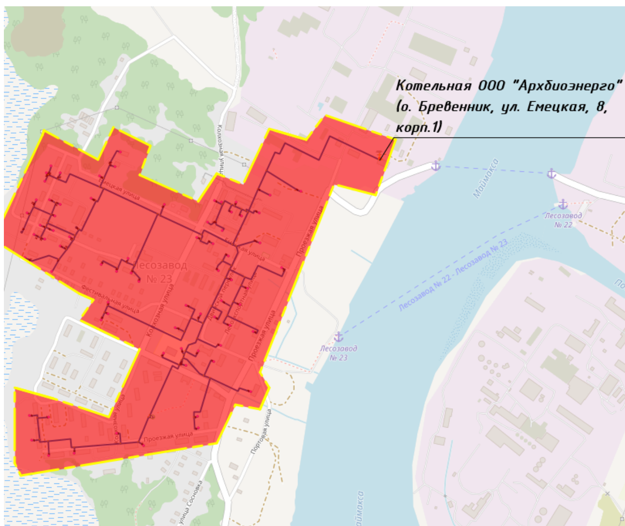
Рисунок 8. Зона действия котельной ООО «Архбиоэнерго» о. Бревенник, ул. Емецкая д. 8, корп.1
