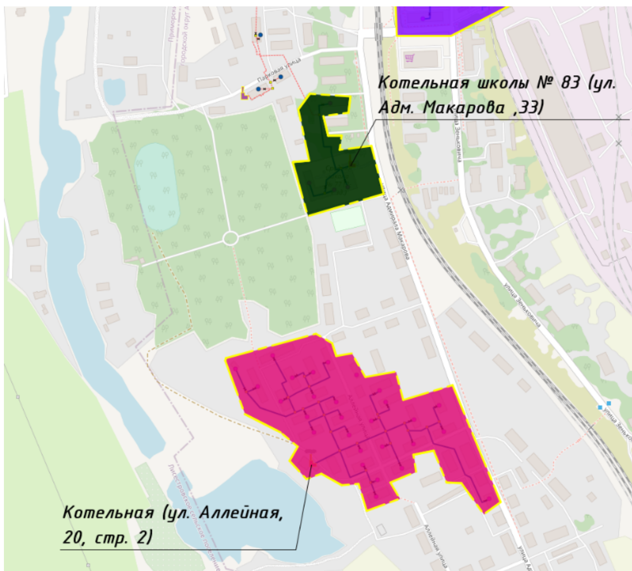
Рисунок 33. Зоны действия котельных ул. Аллейная 20, стр. 2 и котельной школы № 83 ул, Адм. Макарова 33
