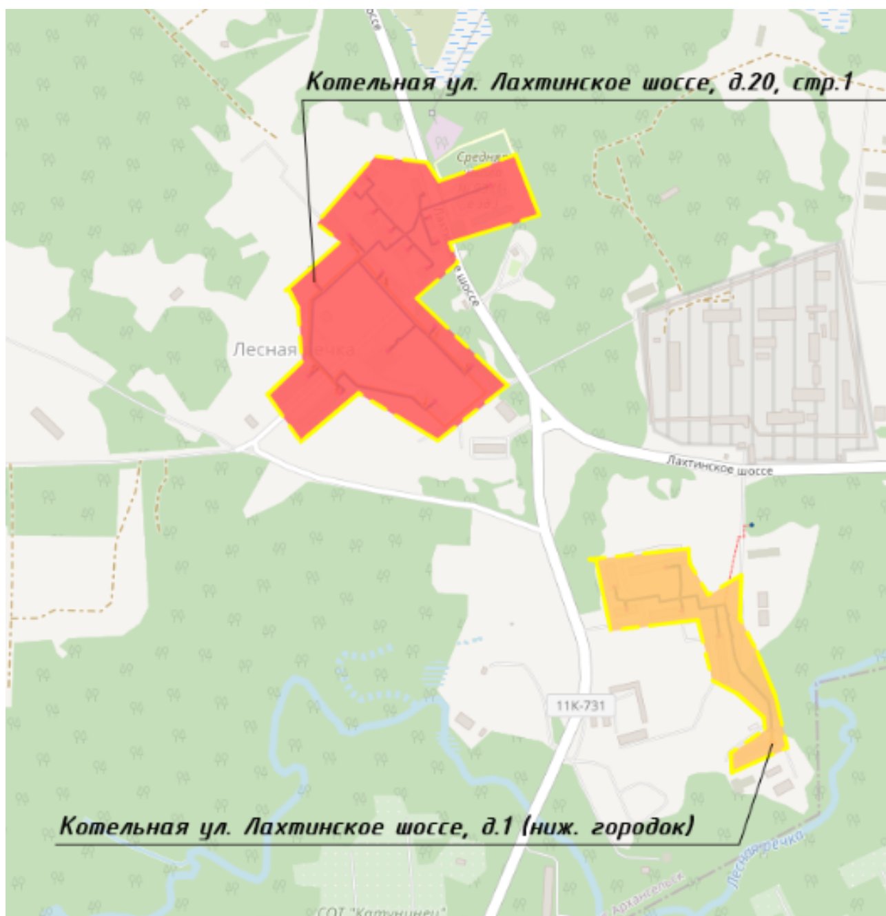
Рисунок 12. Зоны действия котельных ул. Лахтинское шоссе, д. 20, стр. 1 и ул. Лахтинское шоссе, д. 1 (нижний городок)
