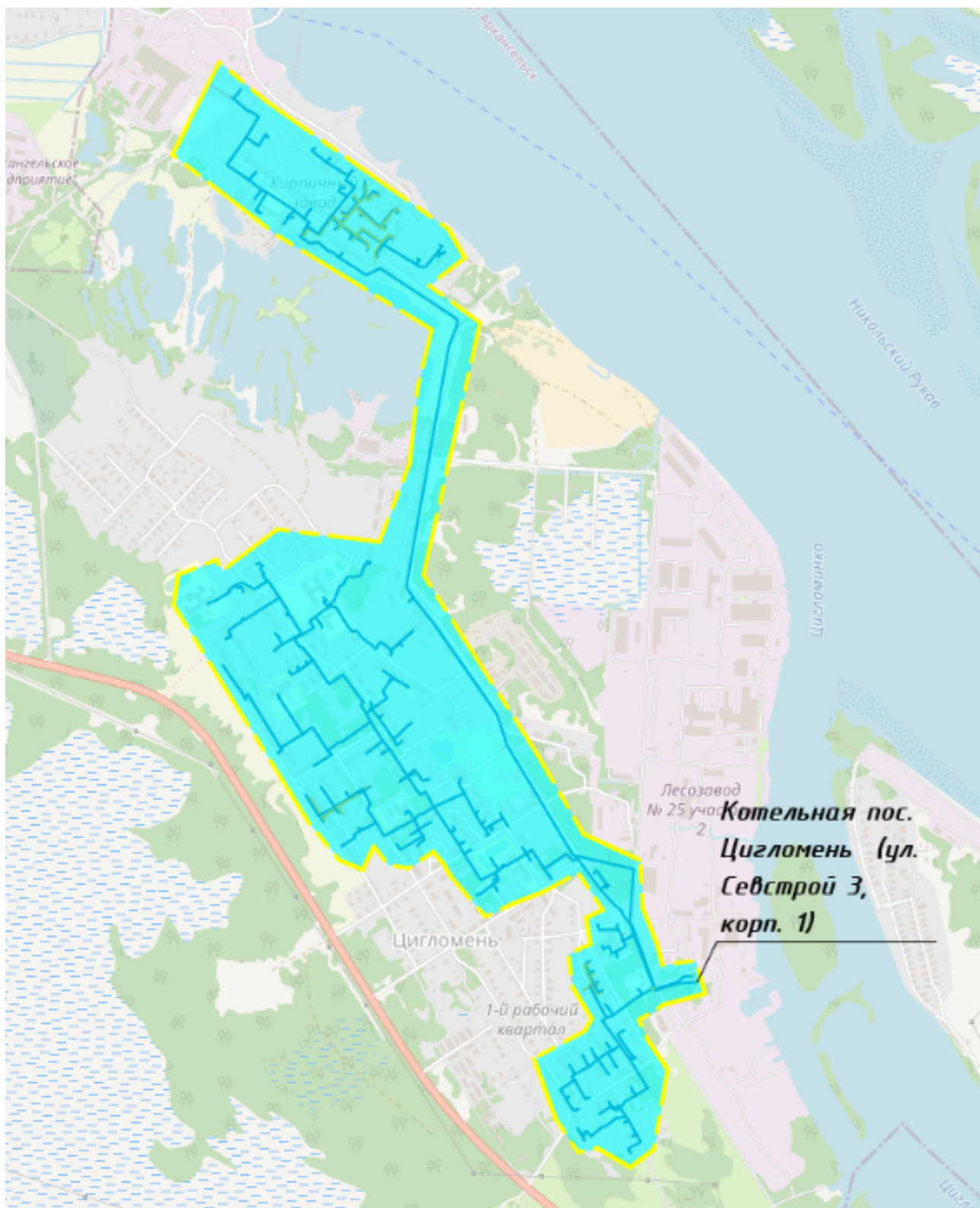
Рисунок 23. Зона действия котельной пос. Цигломень, ул. Севстрой 3, корп. 1
