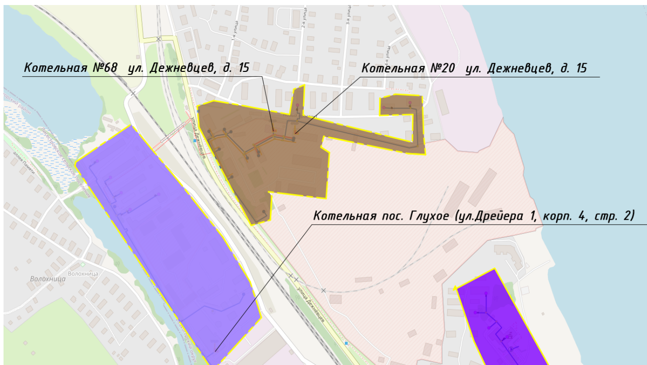
Рисунок 4. Зоны действия котельных ФГБУ «ЦЖКУ» МО России и котельной п. Глухое (ул. Дрейера 1, корп. 4, стр. 2)
