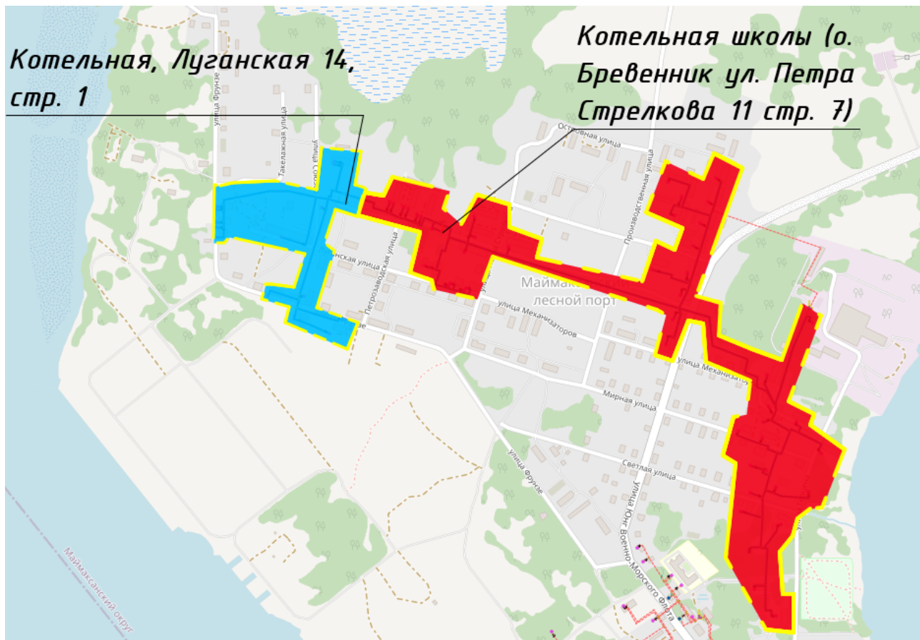
Рисунок 15. Зоны действия котельных ул. Луганская 14, стр. 1 и о. Бревенник, ул. Петра Стрелкова 11, стр. 7
