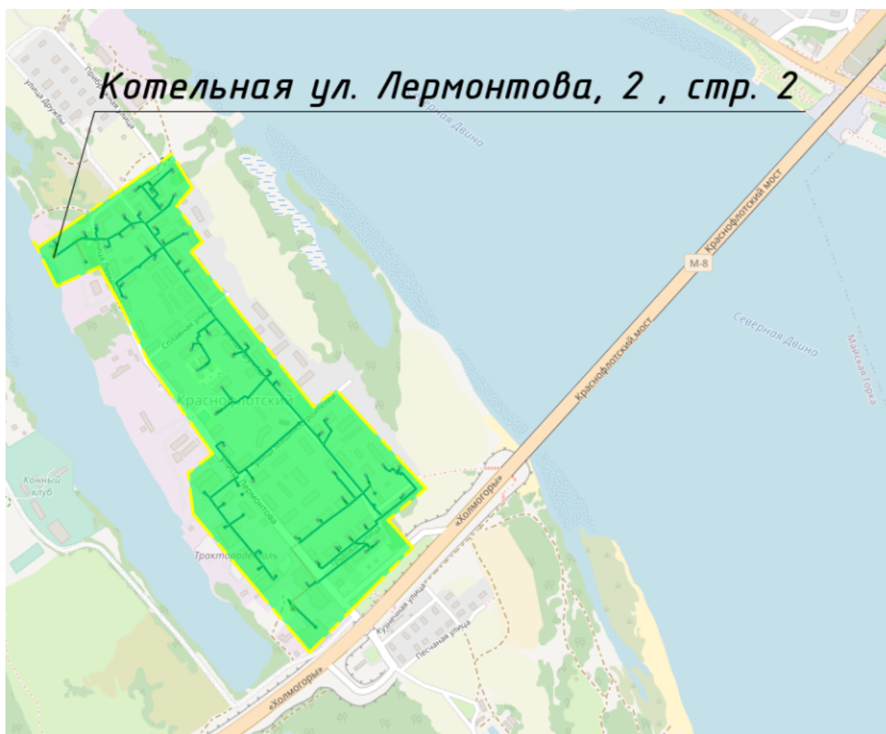
Рисунок 13. Зона действия котельной ул. Лермонтова 2, стр. 2
