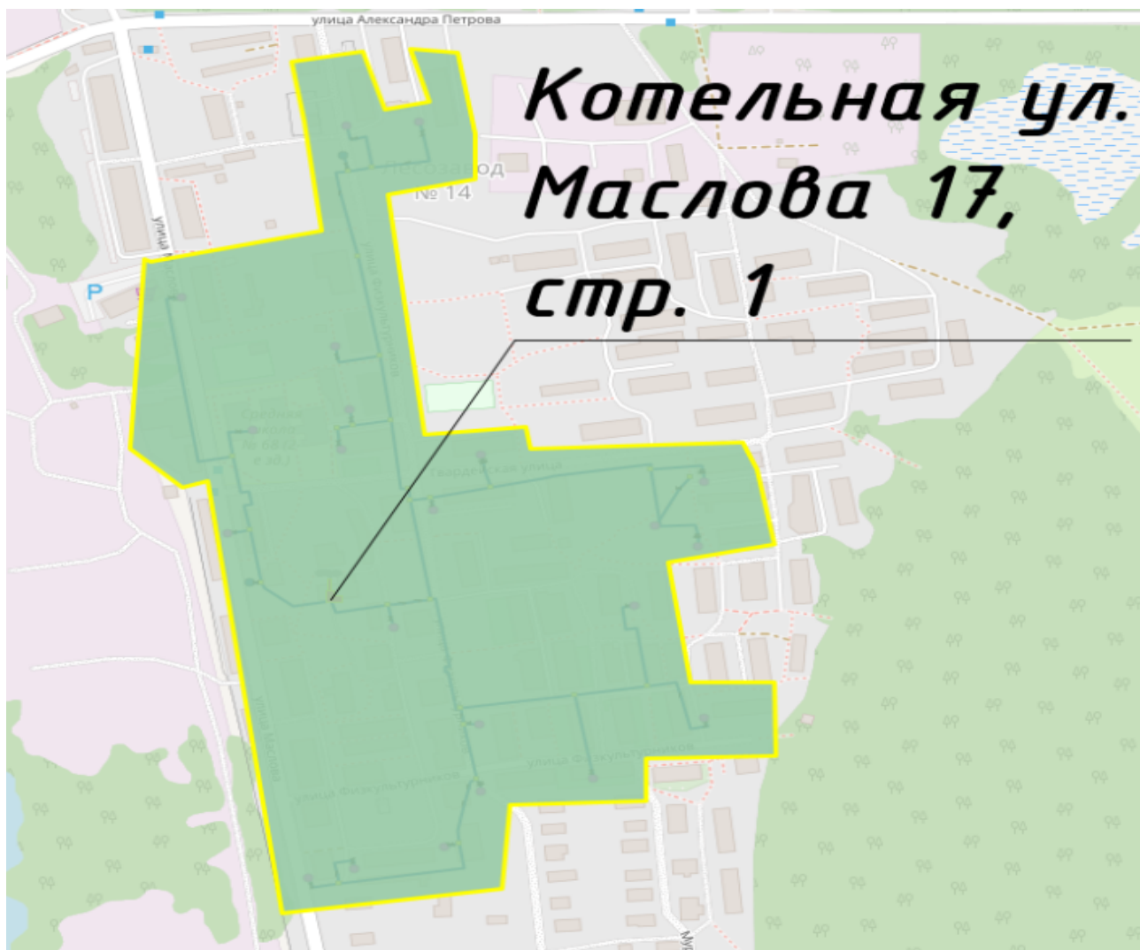
Рисунок 18. Зона действия котельной ул. Маслова 17, стр. 1
